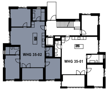
ÜBERSICHT ERDGESCHOSS
